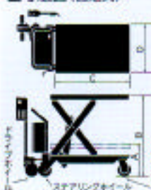
■ 寸法図 (自走式)
